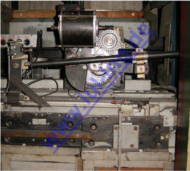
Abb. 1: Otis 9550 vor dem Umbau (hier: TL)
