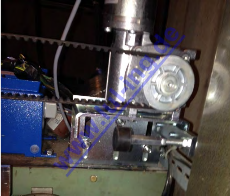
Abb. 8: TSG Antrieb - aufgebaut an Schließeseite
