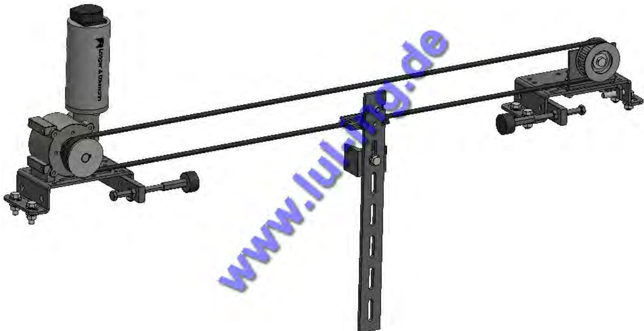
Abb. 2: Schmitt und Sohn Kette Umbau Übersicht
