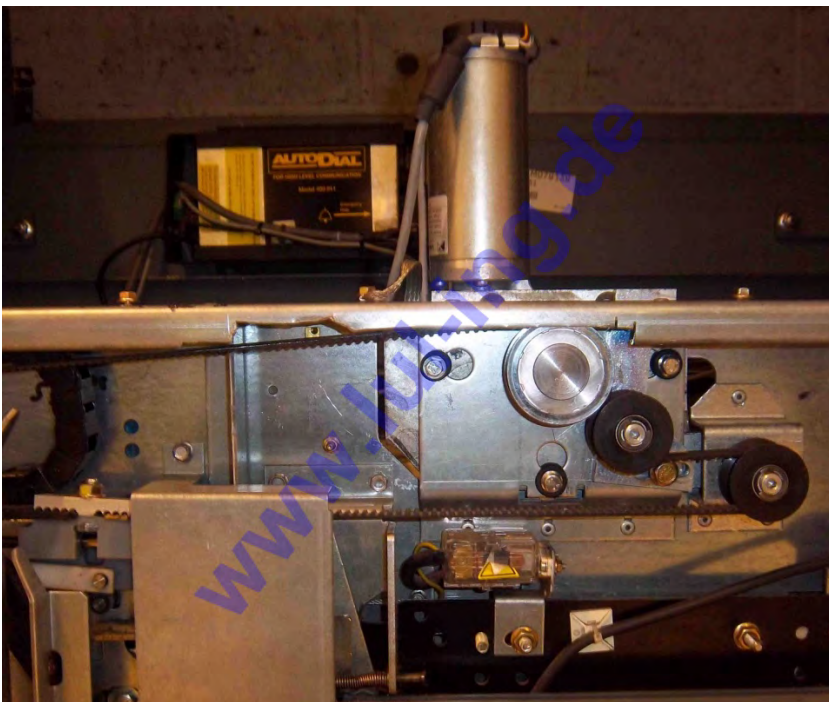
Abb. 2: Thyssen VF11 L&L Umbau
