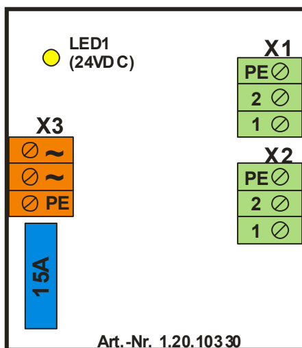
Fig. 5: Électronique du TSG avec platine d'extension pour la commande de la came mobile L&L
