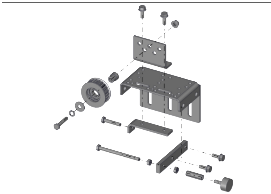
Imagen 12: Montaje de la unidad de inversión
