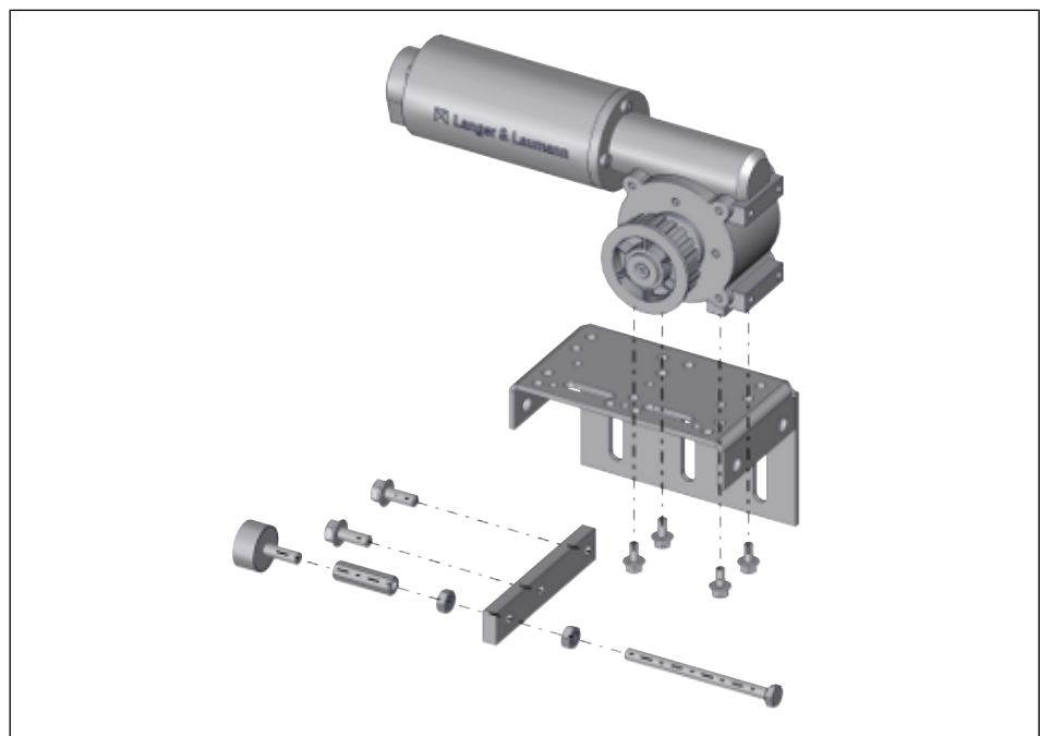
Imagen 14: Montaje de la unidad de accionamiento
