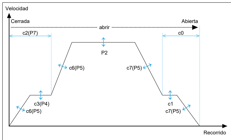
Imagen 21: Curvas de maniobra "Abrir" con parámetros avanzados
