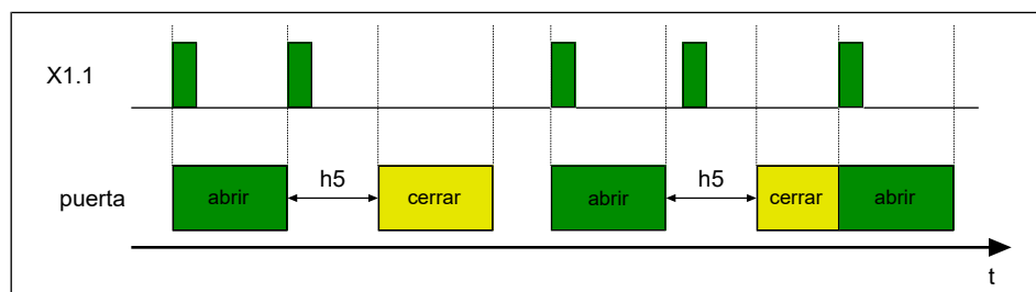
Imagen 11: Secuencia temporal del modo por impulsos (variante 2)
