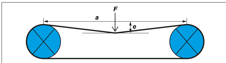
Imagen 16: Determinación de la tensión de la correa dentada
