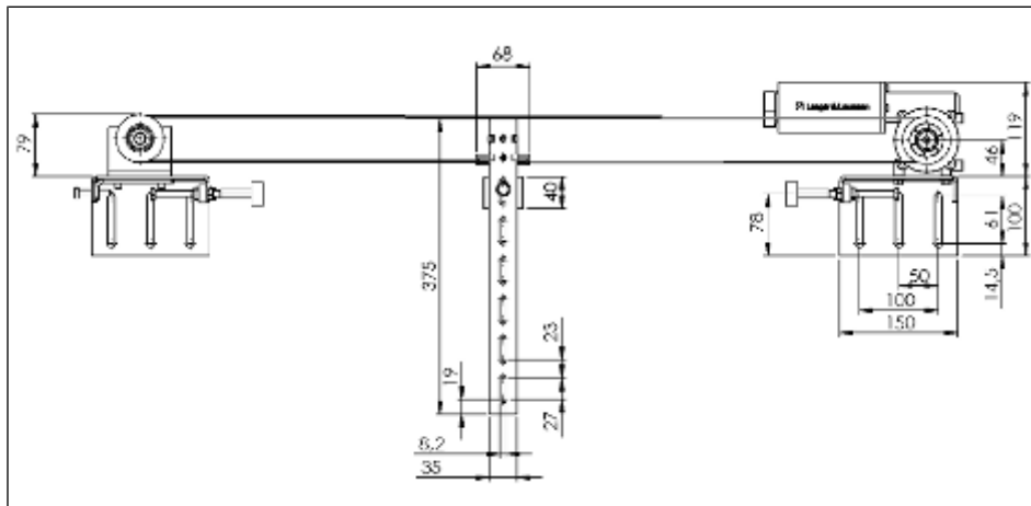
III. 6: Dimensions du mécanisme de l'entraînement de porte (vue de face) (Données en mm)
