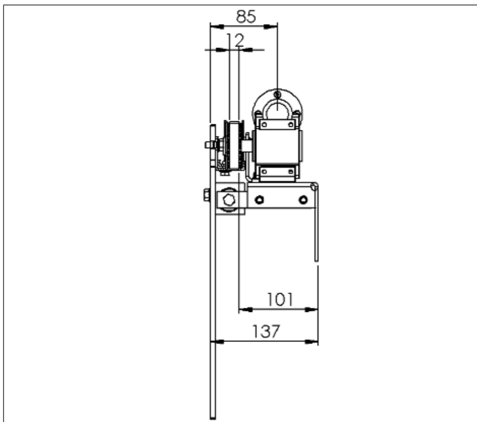
III. 7: Dimensions du mécanisme de l'entraînement de porte (vue de côté) (Données en mm)
