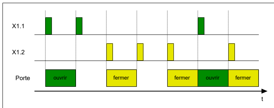
III. 10: Séquence temporelle du mode à impulsions (variante 1)
