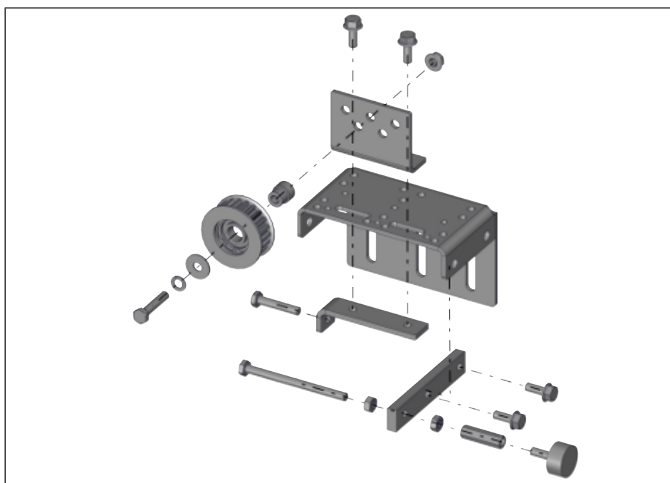
III. 12: Assemblage de l'unité de renvoi
