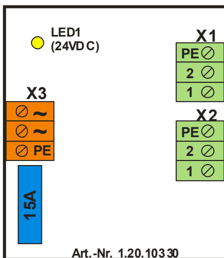
Fig. 4: Électronique du TSG avec platine d'extension pour la commande de la came mobile L&L
