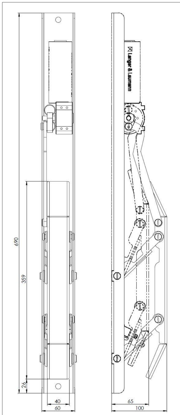
Fig. 3: Came mobile L&L ouverte (position alternative fermée)
