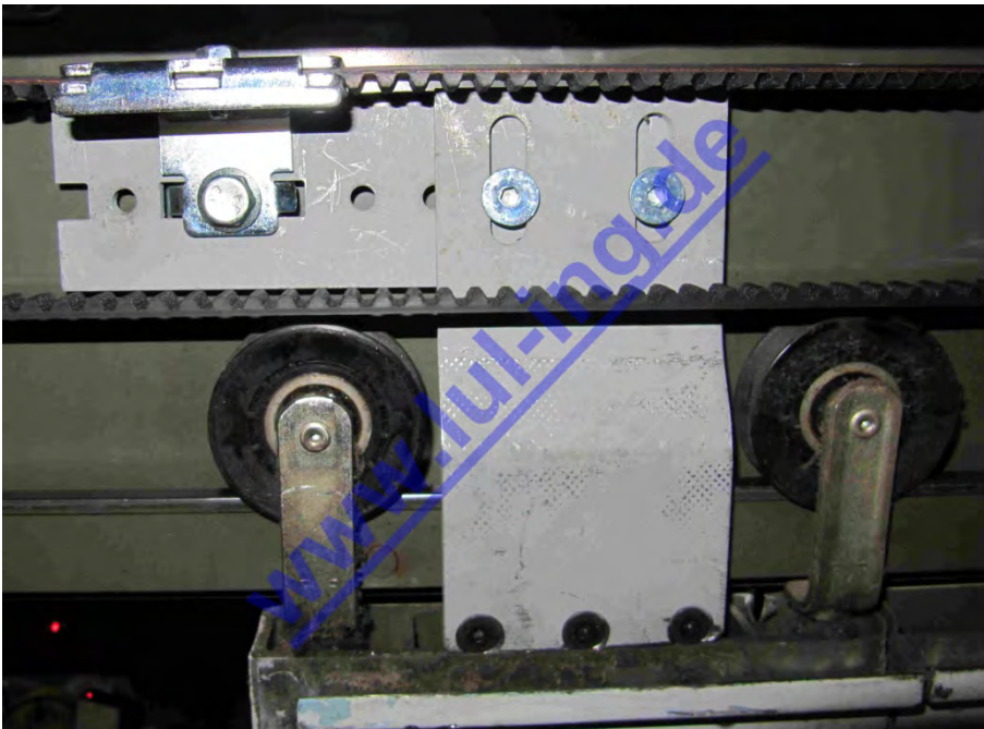
Abb. 6: TSG in Peignen Schachttür - Türflügelmitnehmer
