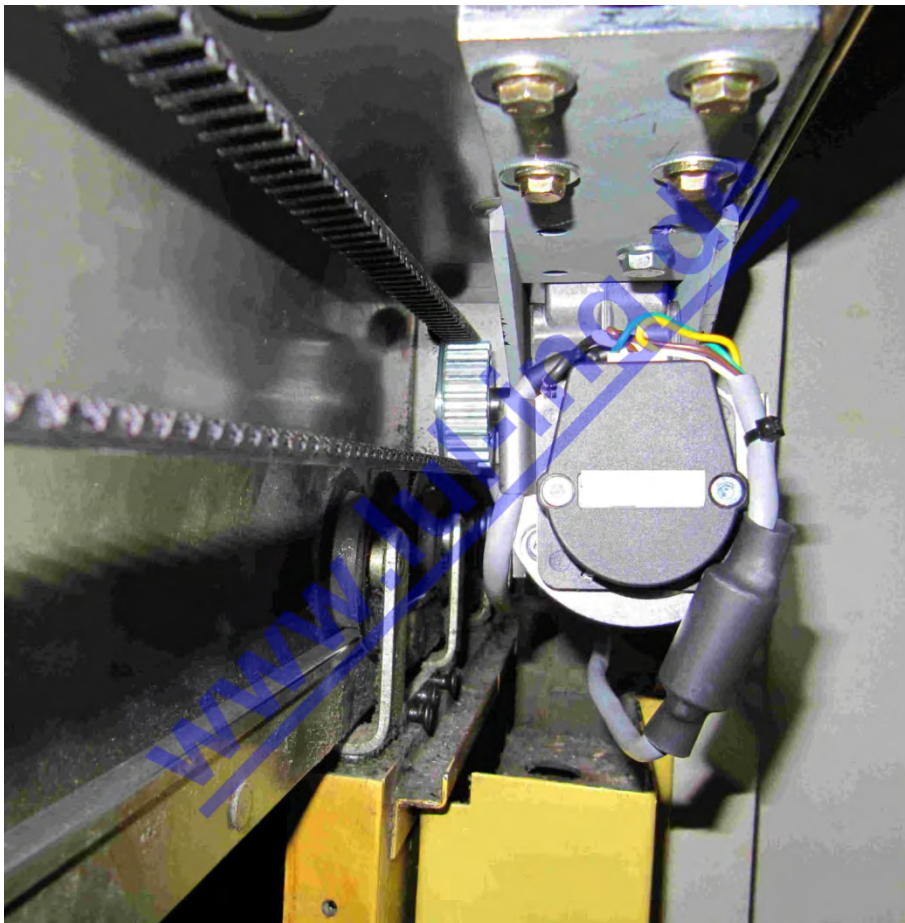
Abb. 4: TSG in Peigen Schachttür - Motorhalterung
