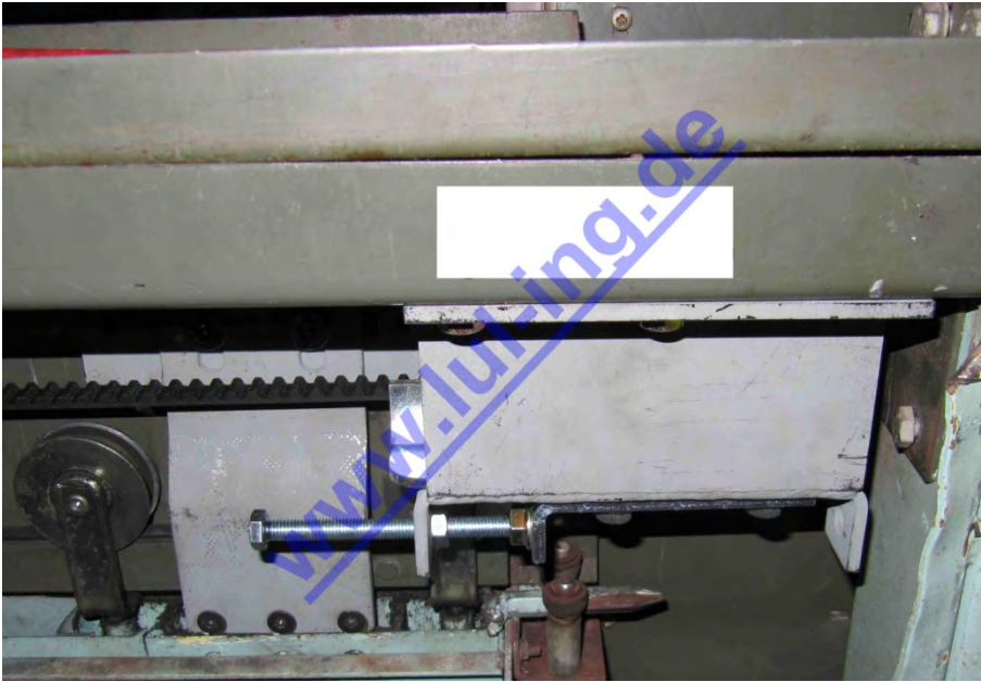
Abb. 10: TSG in Peignen Kabinentür - Halterung Gegenrolle
