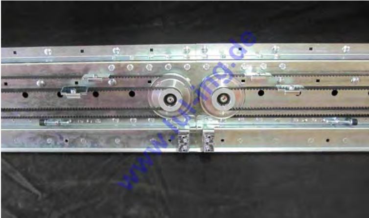
Abb. 7: L&L Türmaschine QKS6 / QKS7 - montierte Mitte
