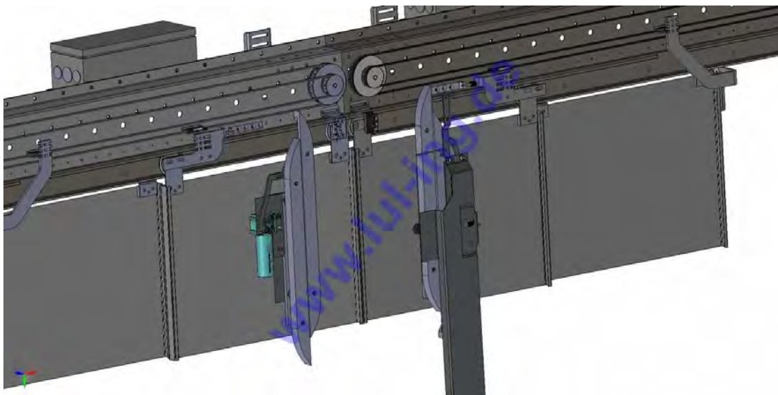
Abb. 6: L&L Türmaschine QKS6 / QKS7 - 3D-Ansicht
