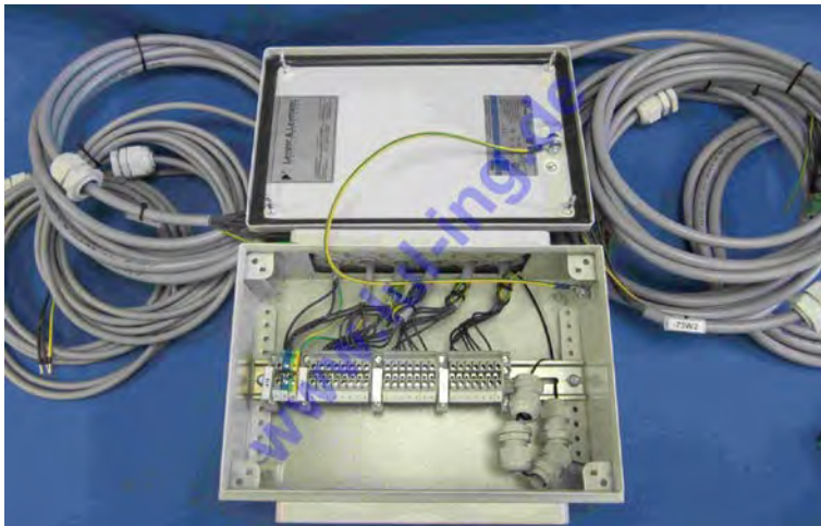
Abb. 14: TSG Anschlusskasten
