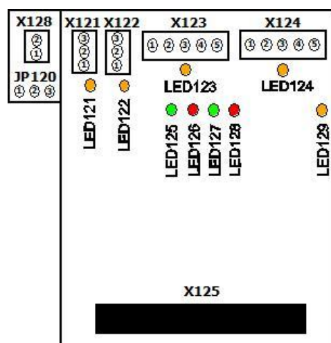
Fig. 8: Module FKTV
