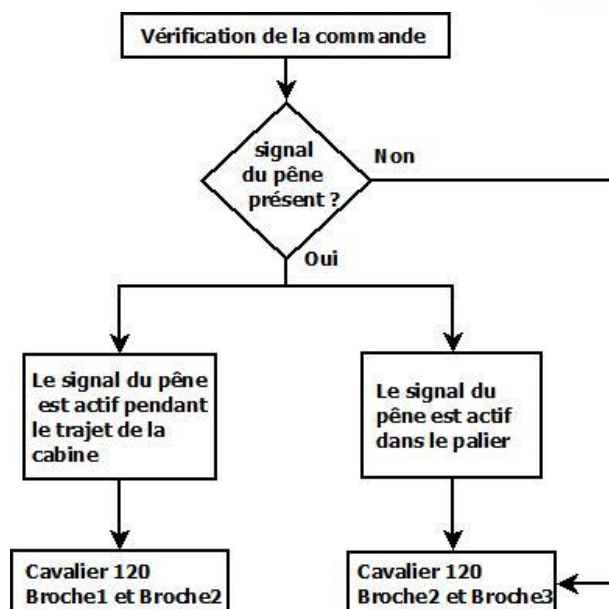
Fig. 7: Organigramme pour le contrôle du signal du pêne et le réglage du cavalier 120
